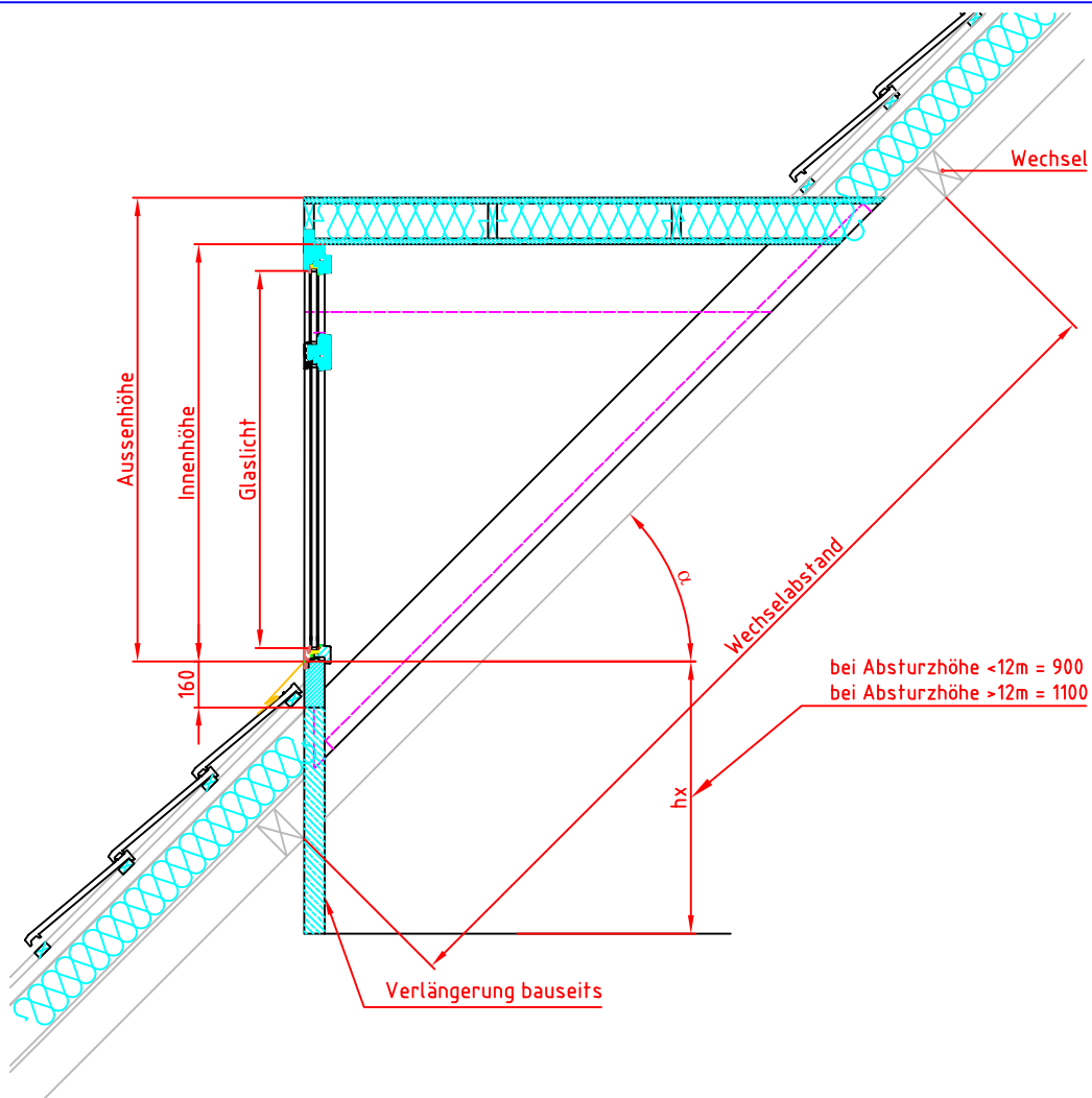
Schnitt B-B
