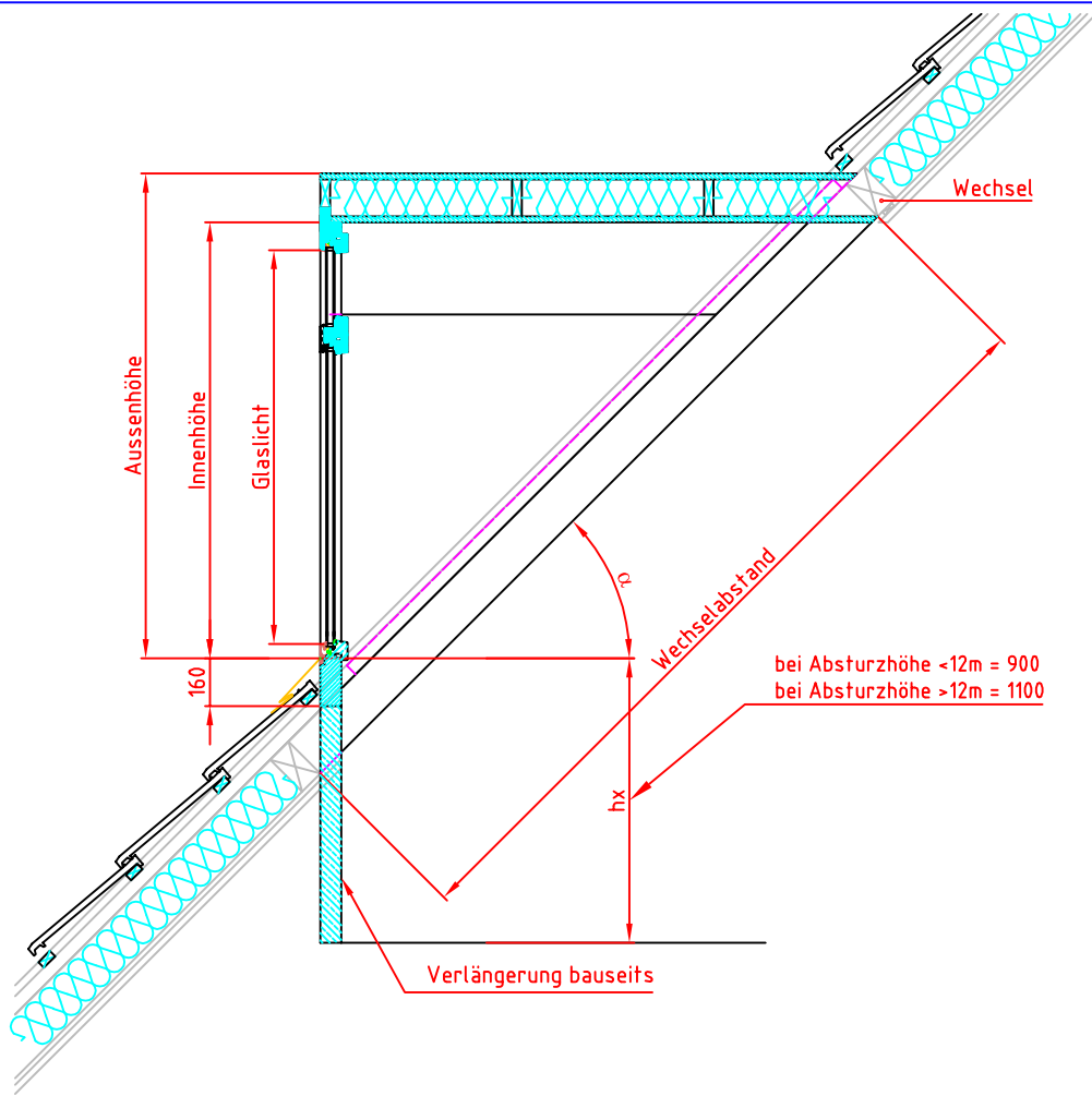
Schnitt B-B
