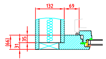
Coupe B-B
