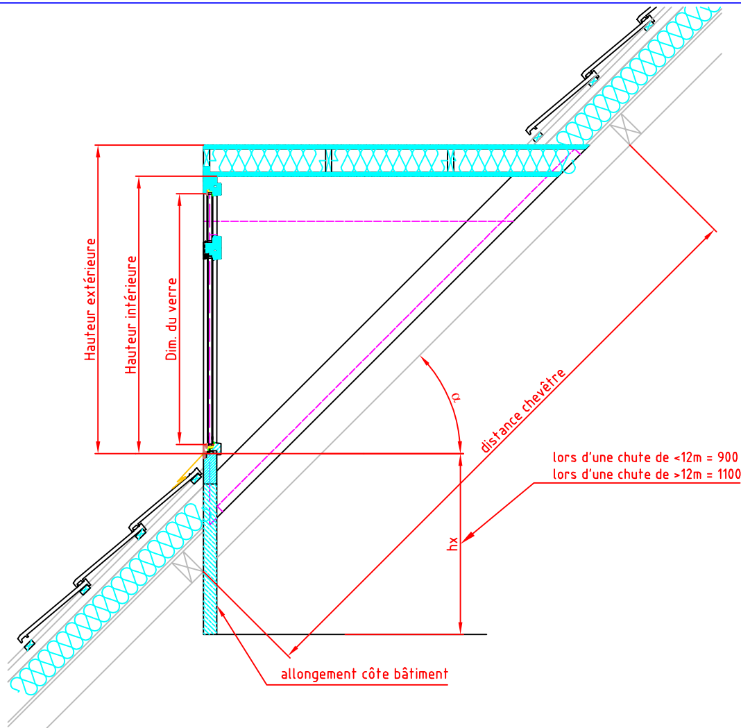
Coupe B-B
