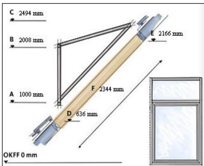
Beispiel: Luxia Pultdachgaube 94 x 101 cm bei 45° Dachneigung
